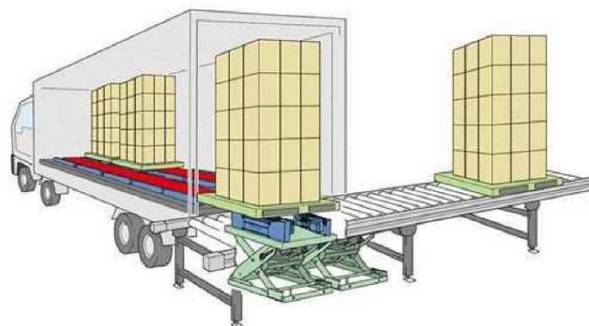
自動積込み・荷下ろしシステム
