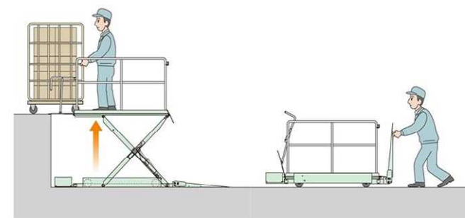
段差解消リフト
